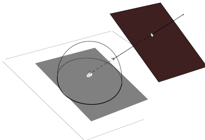
Illustration 5: Principe d'utilisation de l'hémisphère transparent.
