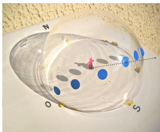
Illustration 4: Course du Soleil relevée sur une demi-sphère transparente. La position indiquée en pointillés correspond au midi solaire.
