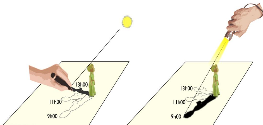
Illustration 3 : Relevé d'ombre portée à l'aide d'une figurine.
