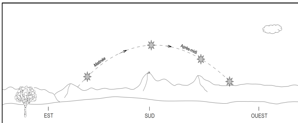
Illustration 1: Exemple de relevé de la course du Soleil, à différents moments d'une journée d'hiver.
