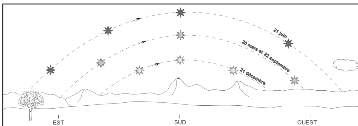
Illustration 1: Relevés des positions du Soleil à différentes dates de l'année.
