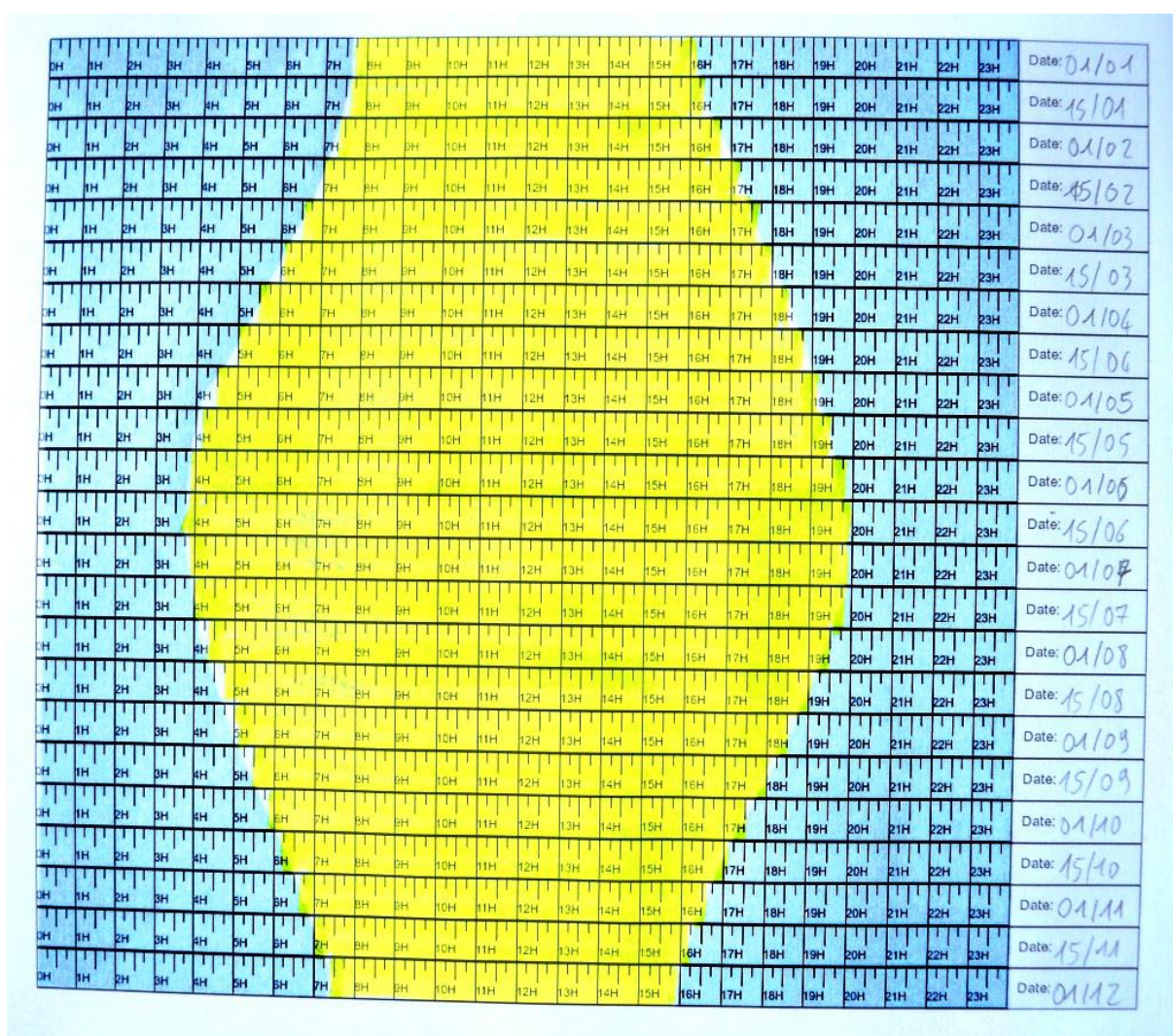
Illustration 5: Assemblages de bandelettes montrant l'évolution au cours de l'année de la durée du jour (en jaune) et de la nuit (en bleu), à Tarbes, selon le tableau des heures en Temps Universel.
